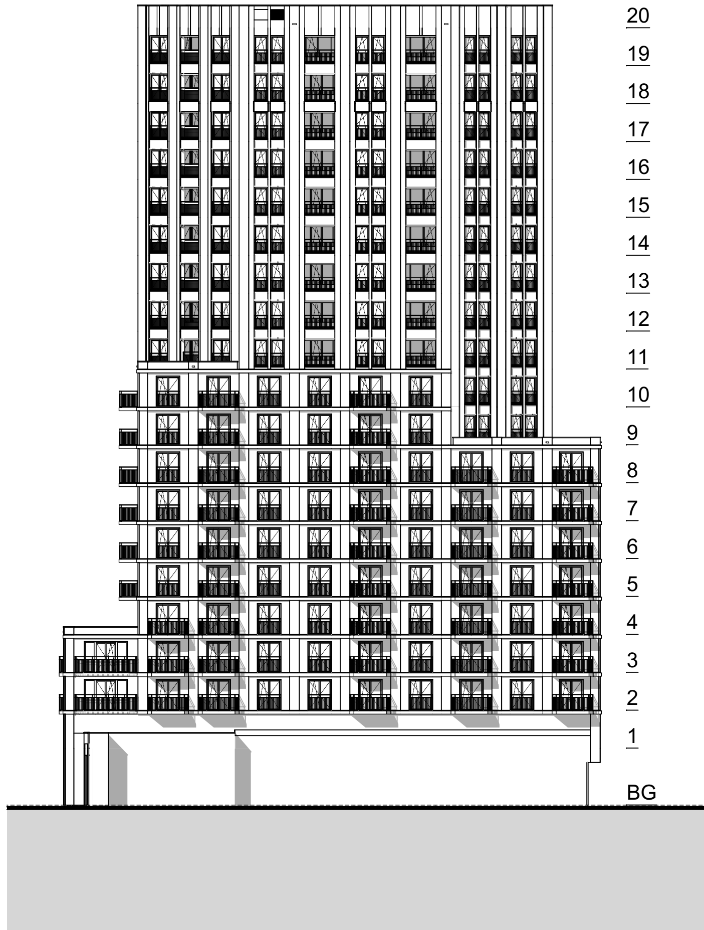
rechtergevel (west)
