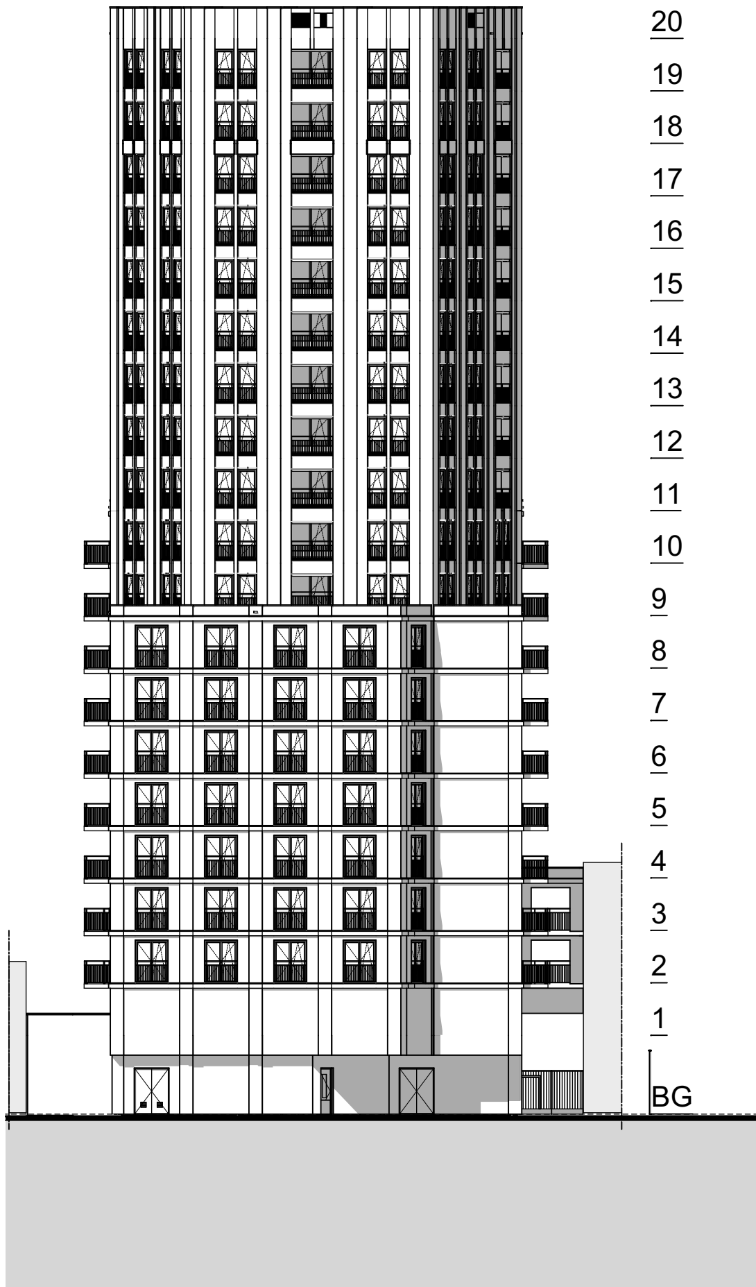
achtergevel (zuid)
