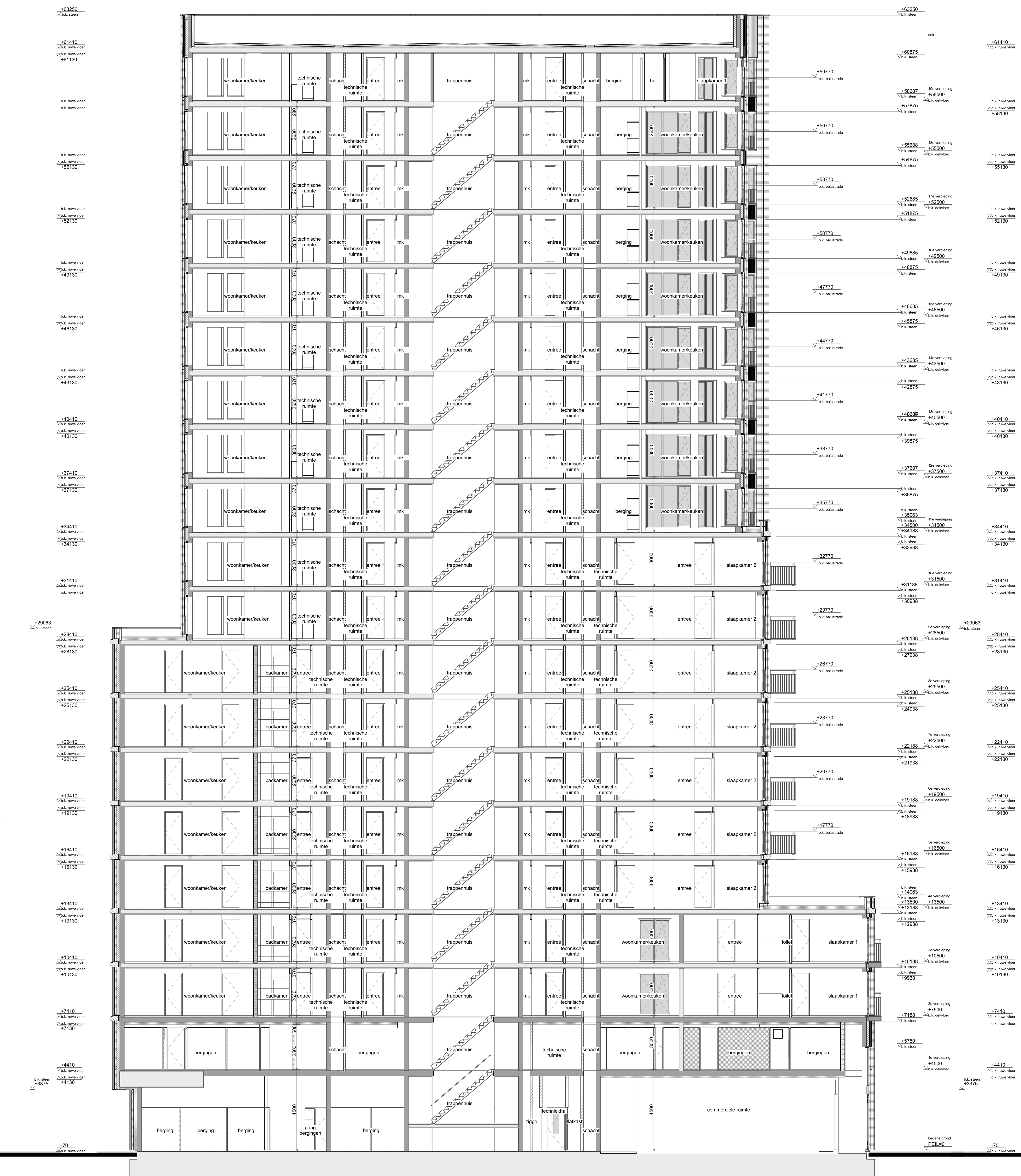
DOORSNEDE A-A
