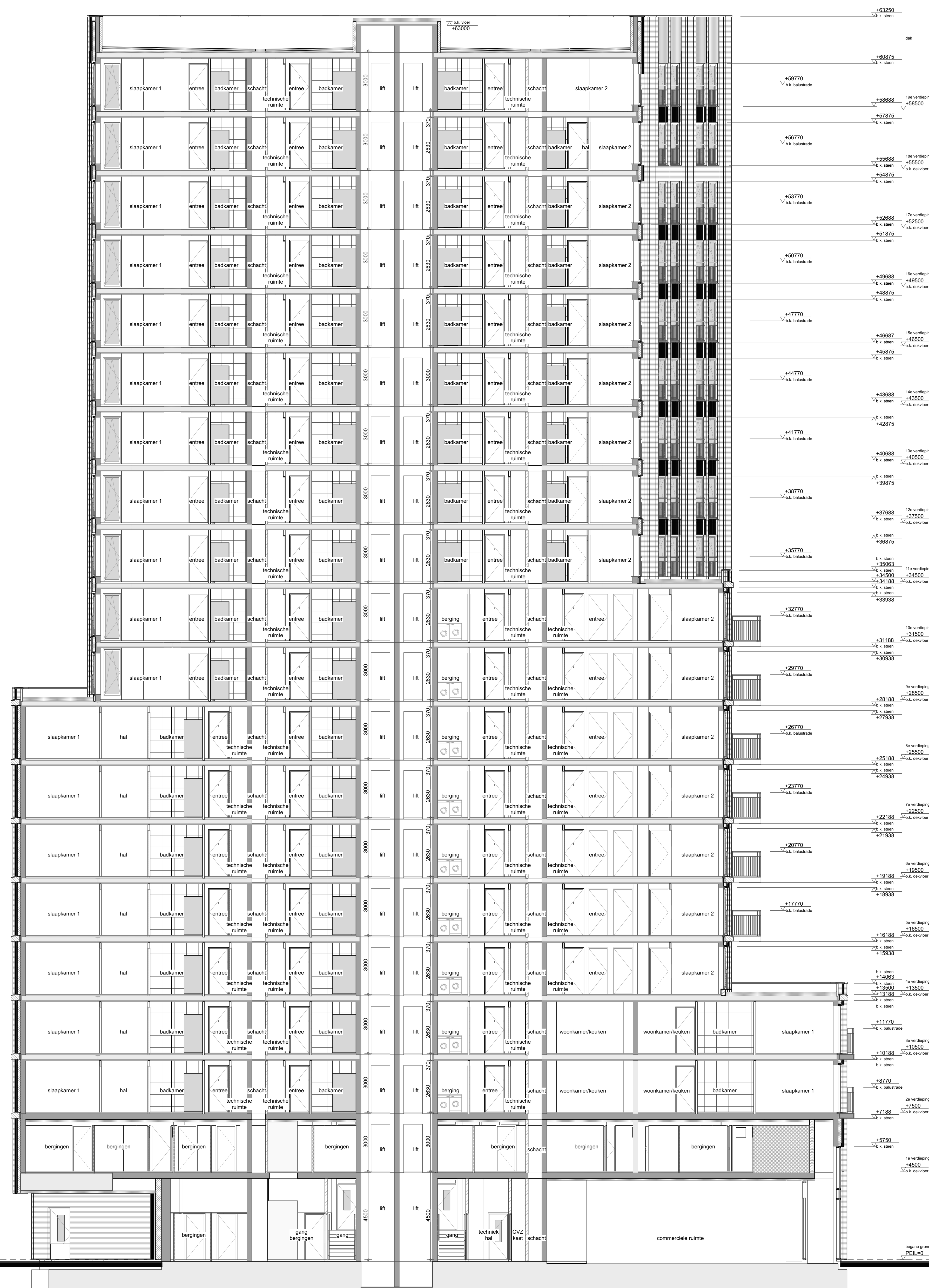
DOORSNEDE B-B
