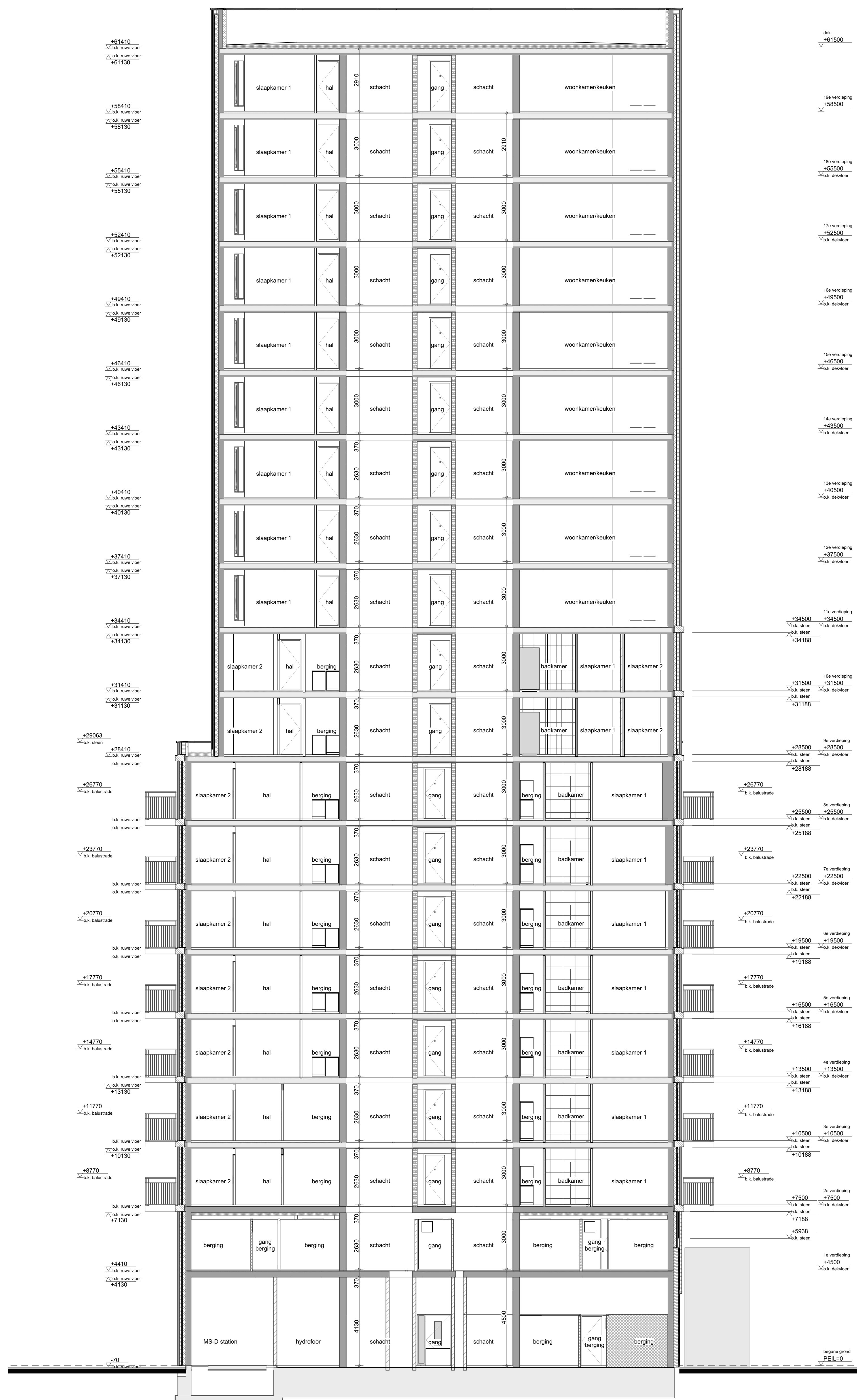
DOORSNEDE E-E
