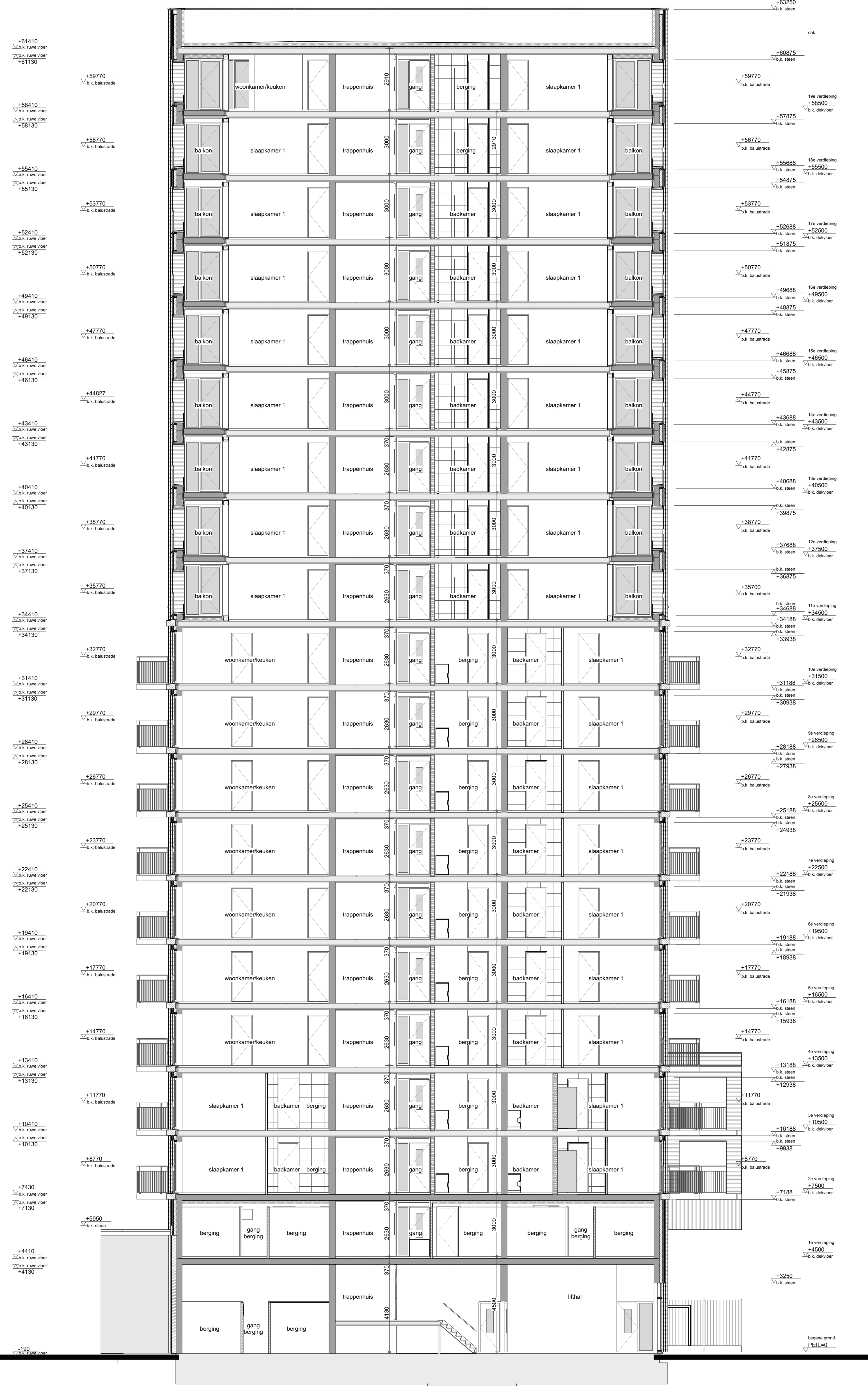
DOORSNEDE F-F
