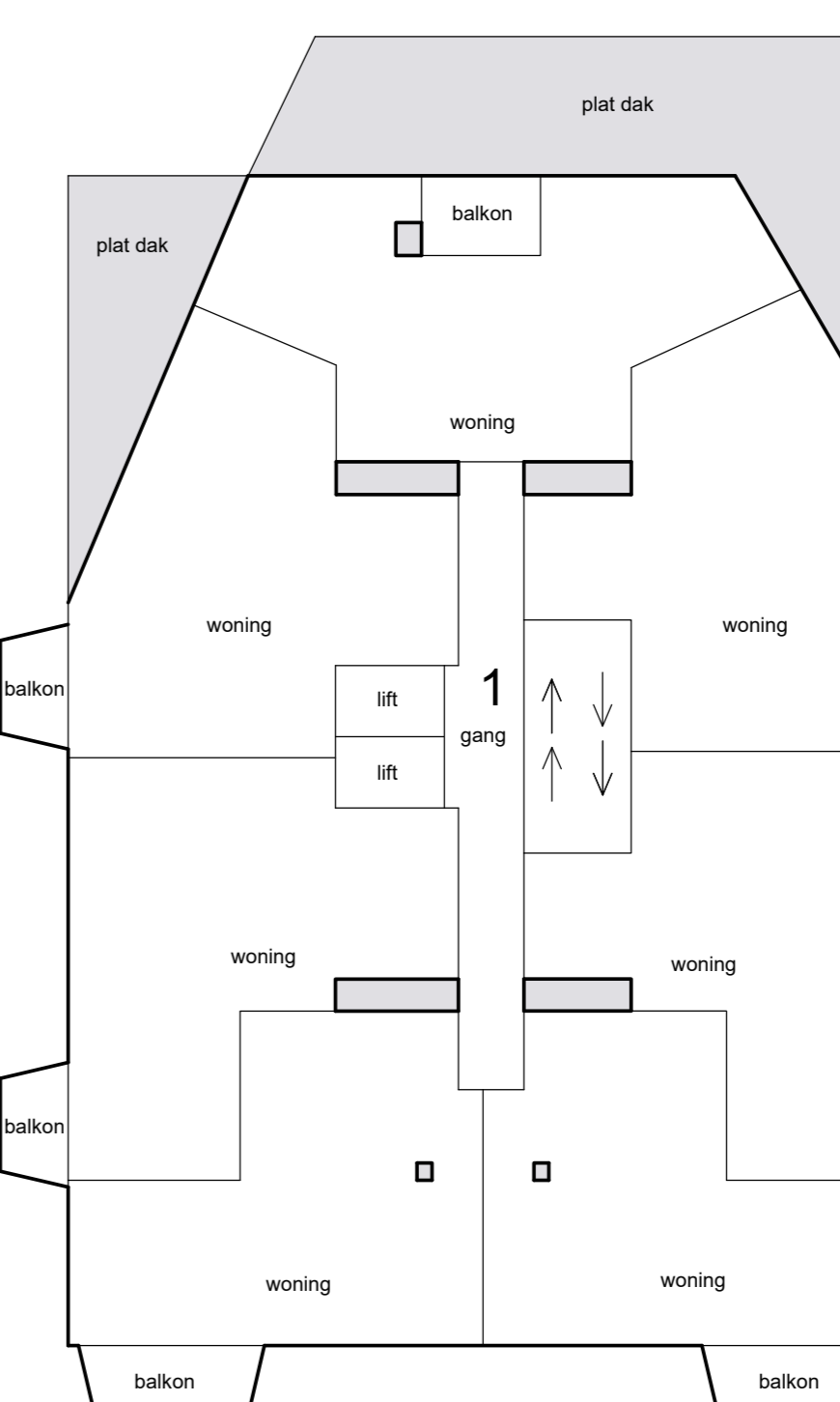
10e etage
