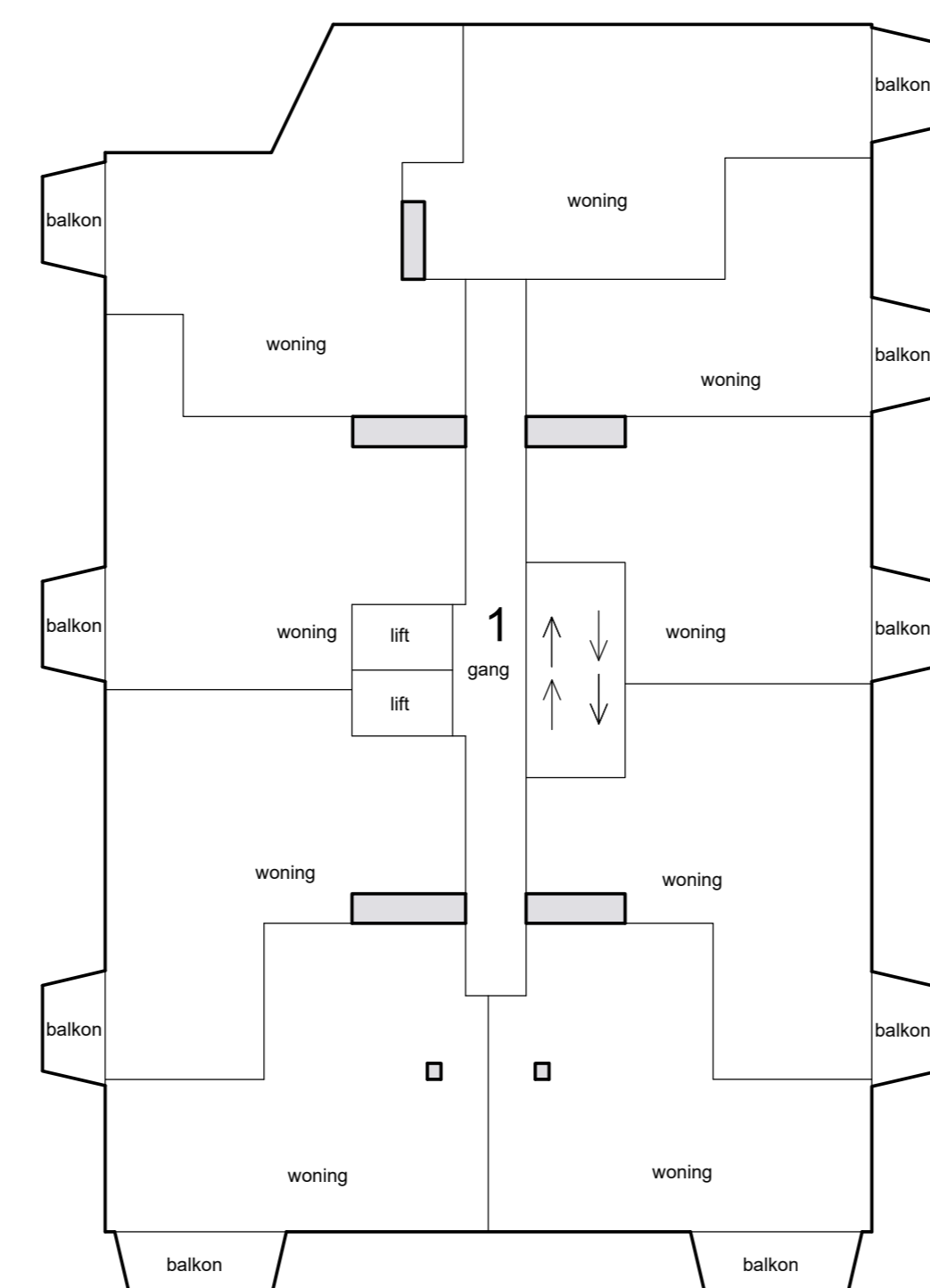
5e etage
