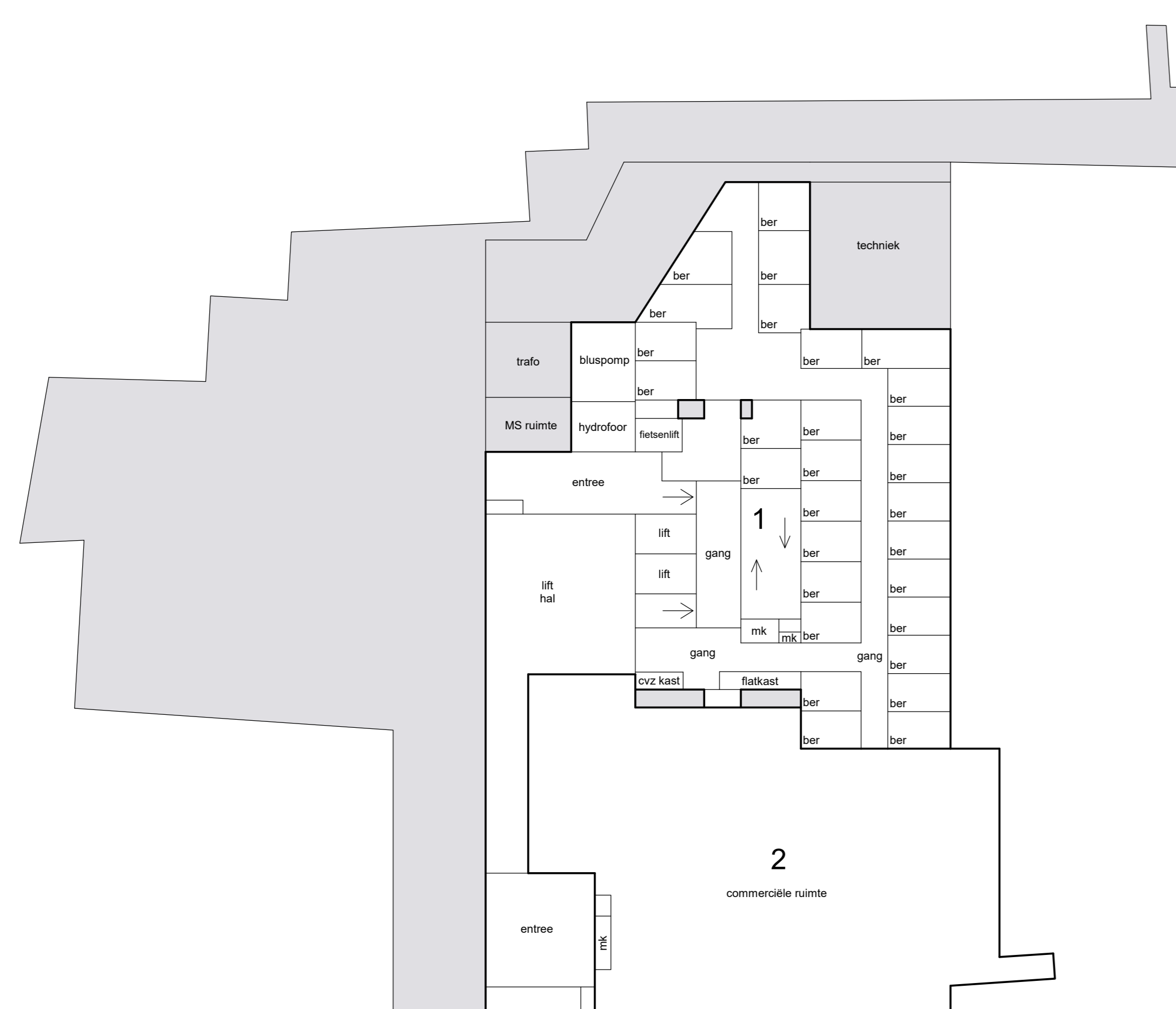
begane grond
