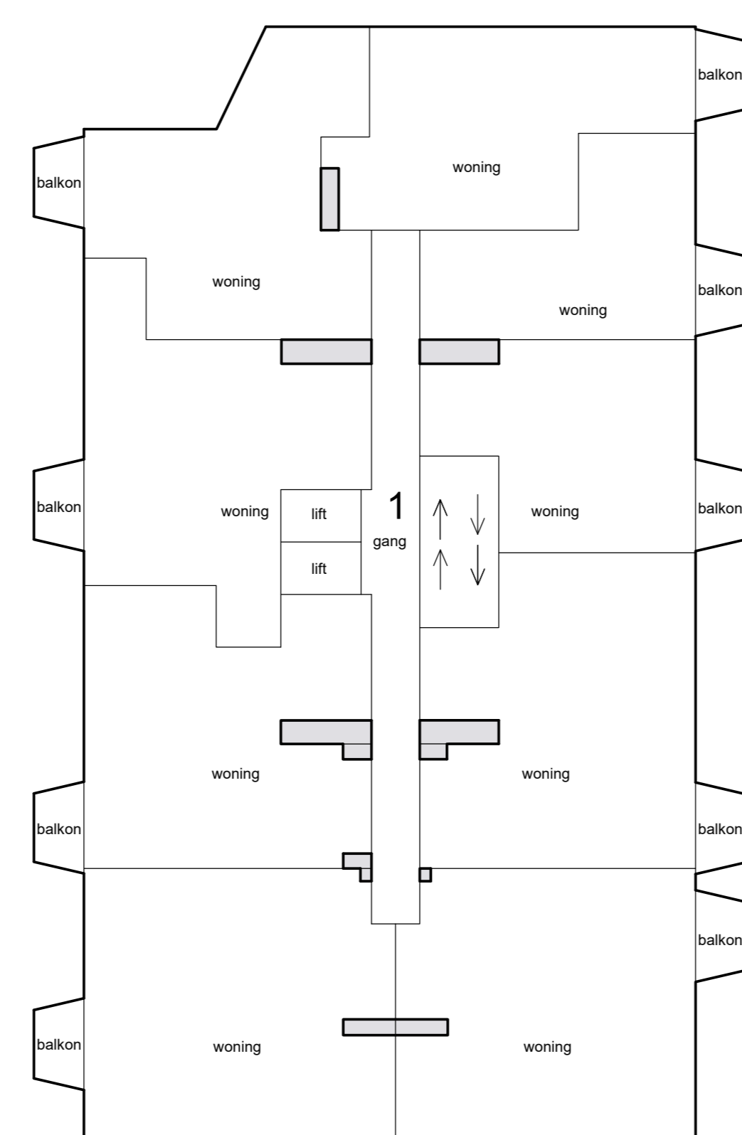
3e etage
